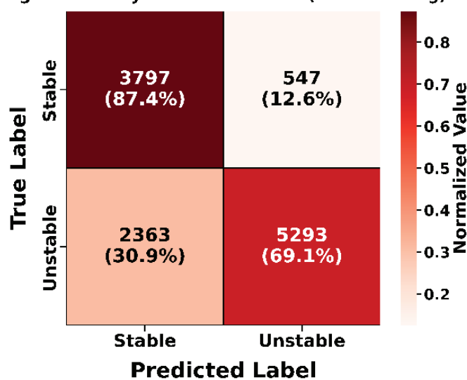
(d) OOF-Stacking
