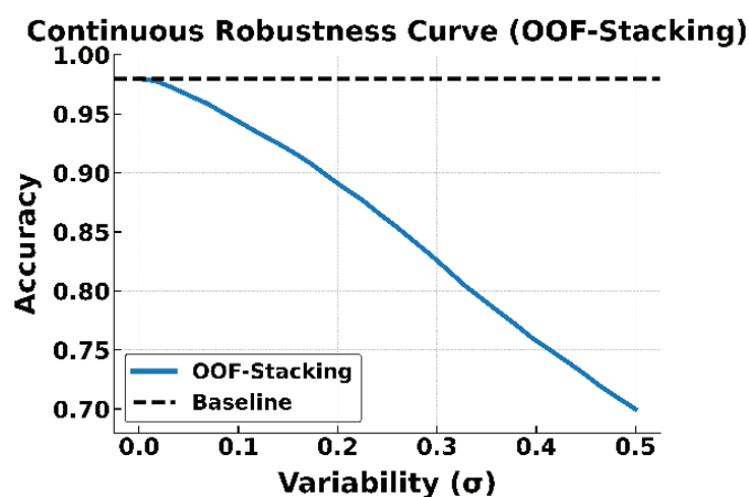
(d) OOF-Stacking
